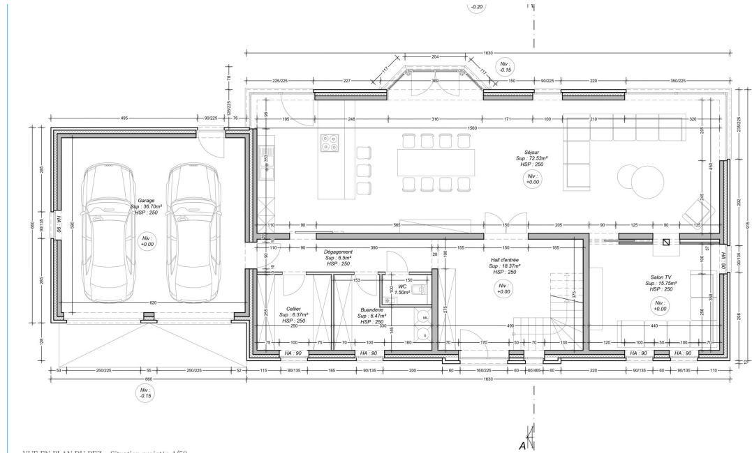
VUE EN PLAN DU REZ – Situation projetée 1/50
